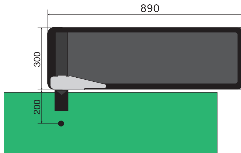
■ 平面图
