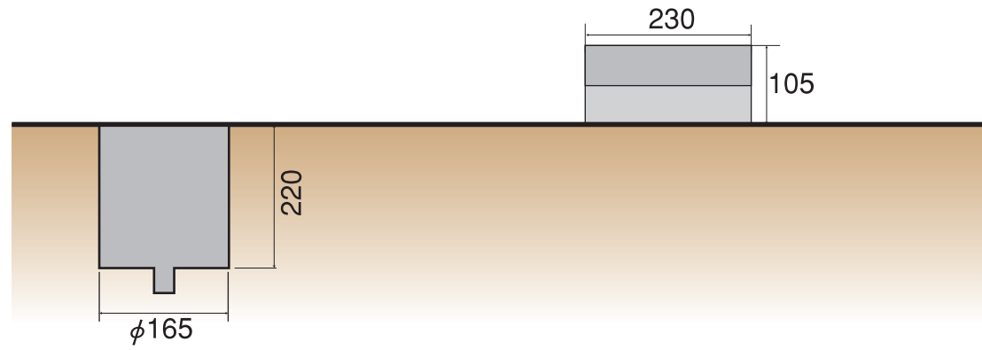
■ 正面図
